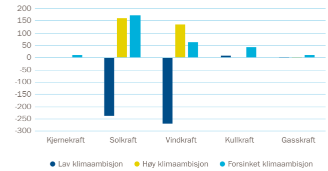
27 Endringer i utbygd kapasitet (GW) i kraftsektoren i Europa for ulike klimaambisjoner i forhold til Lavutslippsscenarioet
